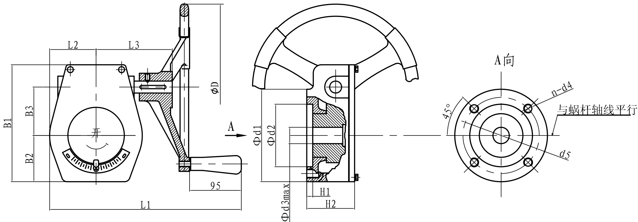
VGC1、3、8外形及连接尺寸
